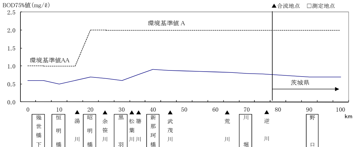
図2-5 那珂川の水質流程変化(BOD75%値)
