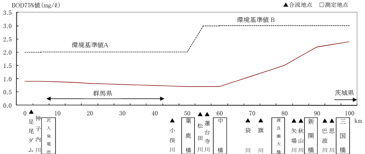
図2-7 渡良瀬川の水質流程変化(BOD75%値)
