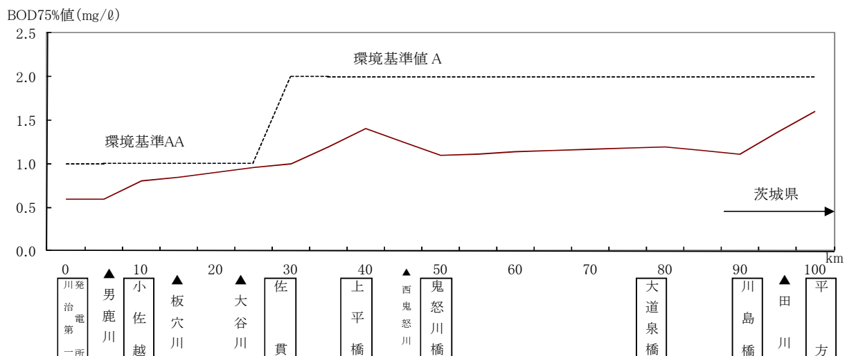
図2-6 鬼怒川の水質流程変化(BOD75%値)
