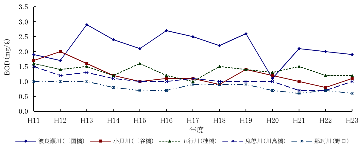
図2-4 主要河川県内末流地点におけるBOD(年平均値)の経年変化
