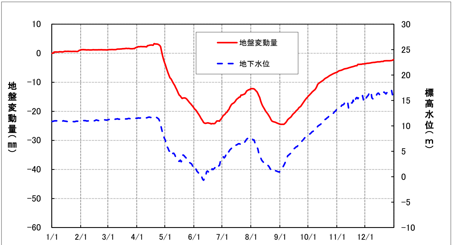
図-3 野木(環境)における地盤変動量及び地下水位状況(令和2(2020)年)
