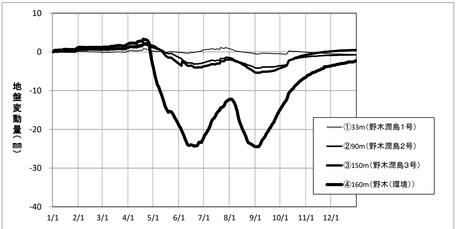
図-4 野木(環境)及び野木潤島における井戸深度別地盤変動量(令和2(2020)年)
