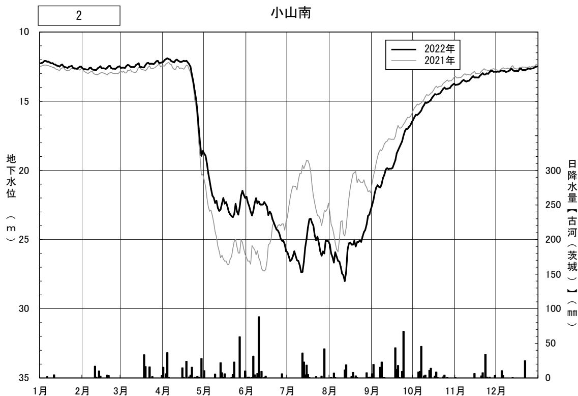
図4.3(6) 日地下水位の年間変動（小山南）
