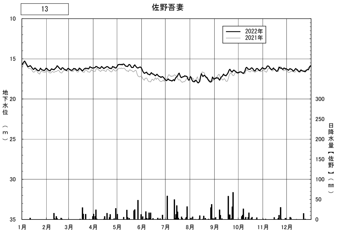
図4.3(24) 日地下水位の年間変動 (佐野吾妻)
