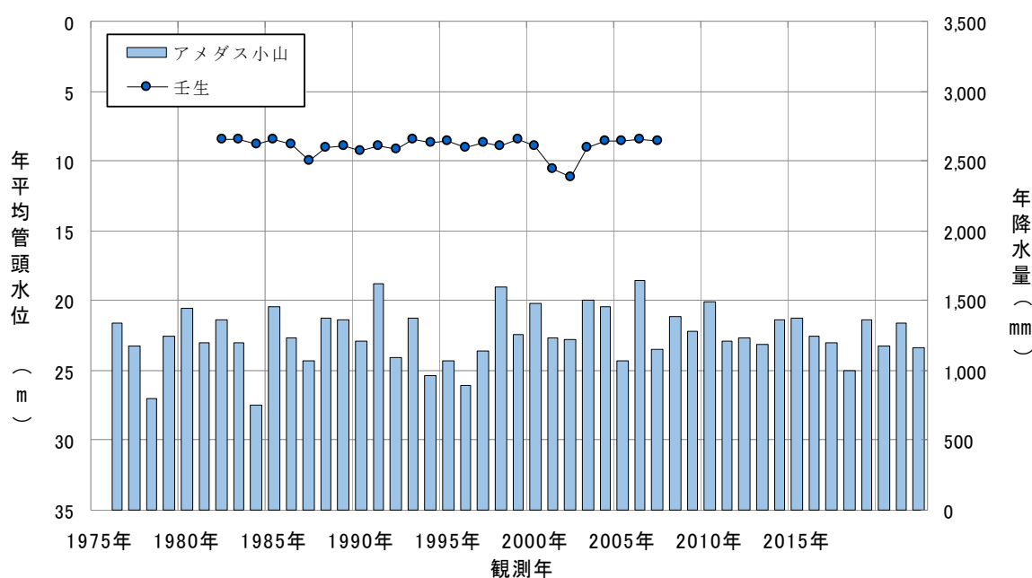
図4.3(68) 年平均地下水位の経年変化（壬生）
