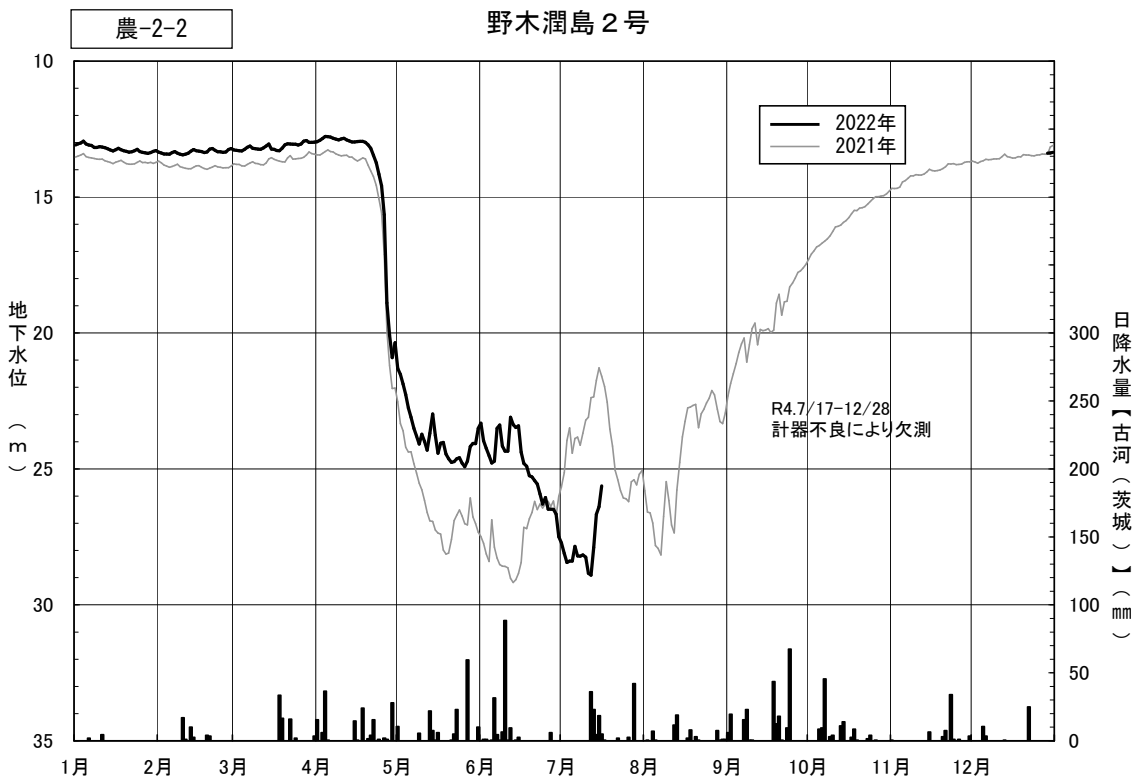
図4.3(52) 日地下水位の年間変動（野木潤島2号）
