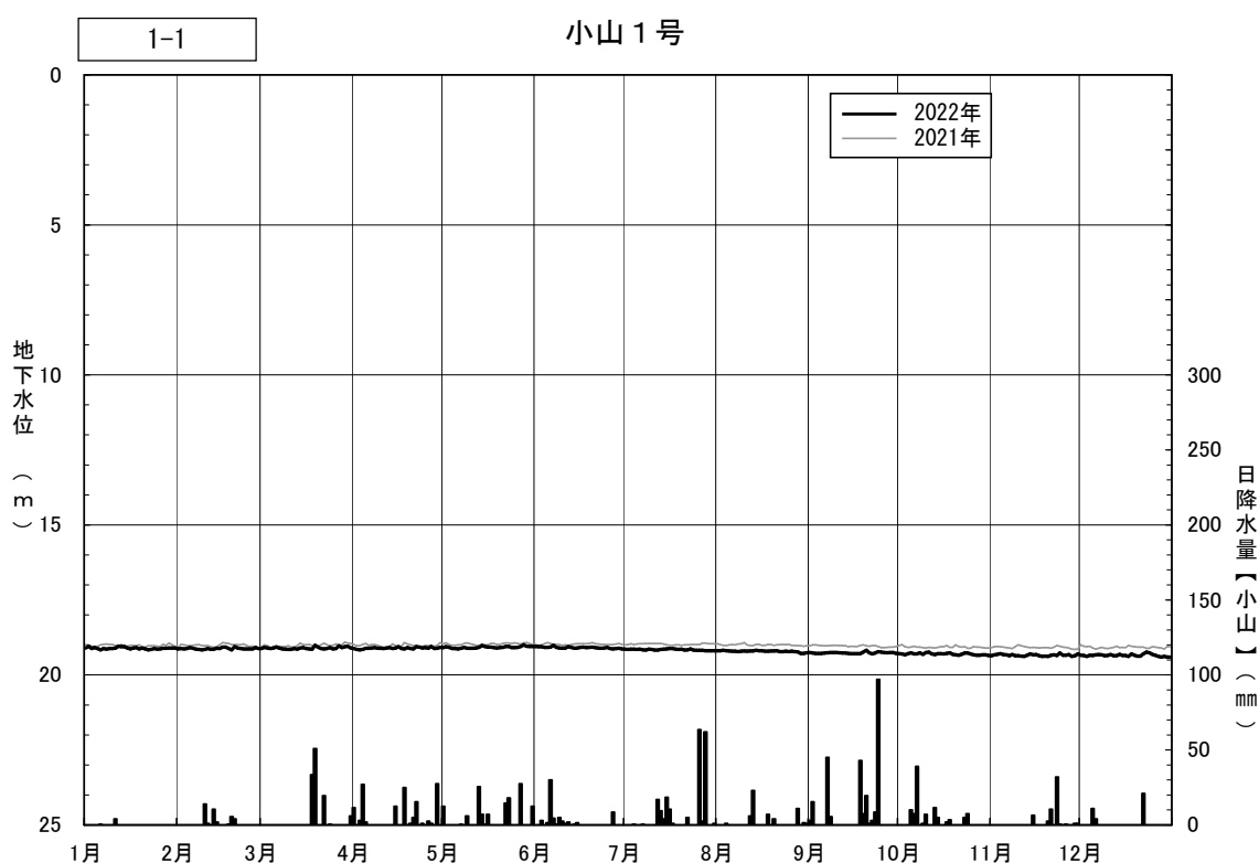
図4.3(2) 日地下水位の年間変動（小山1号）
