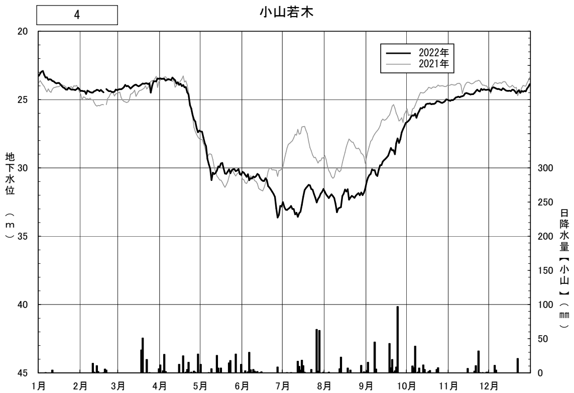
図4.3(9) 日地下水位の年間変動（小山若木）
