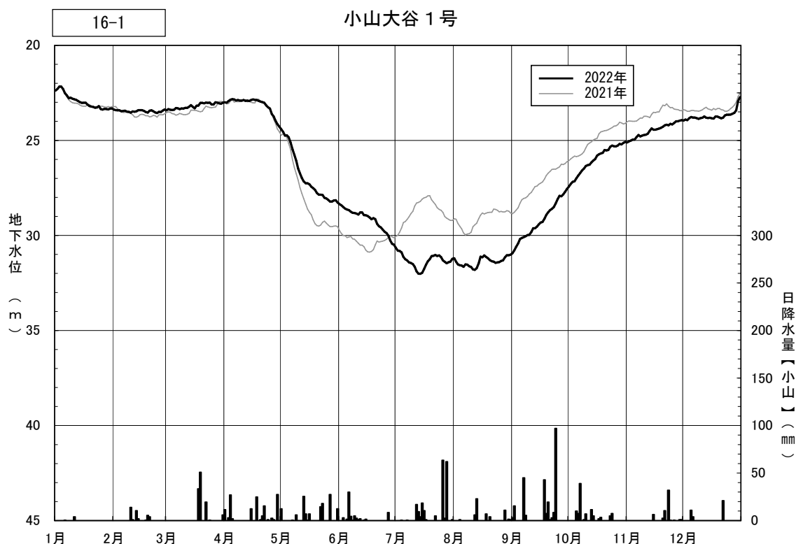
図4.3(30) 日地下水位の年間変動（小山大谷1号）
