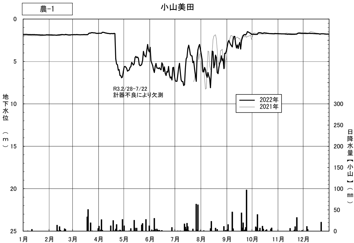
図4.3(48) 日地下水位の年間変動（小山美田）
