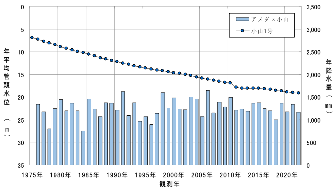
図4.3(1) 年平均地下水位の経年変化（小山1号）
