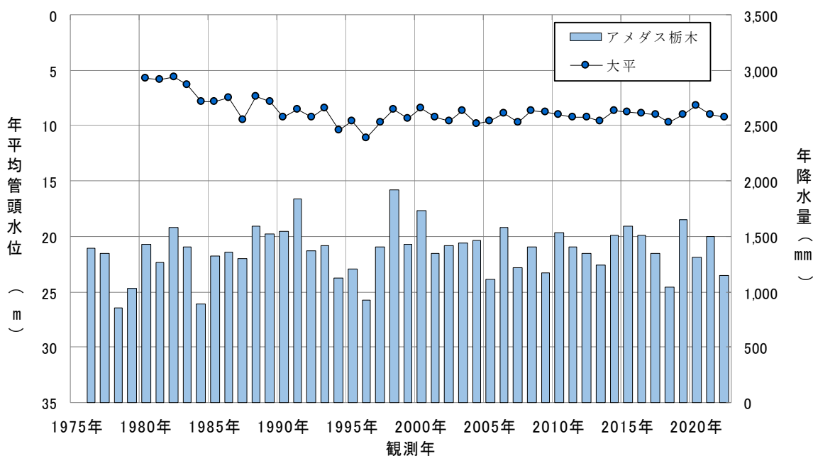
図4.3(14) 年平均地下水位の経年変化 (大平)
