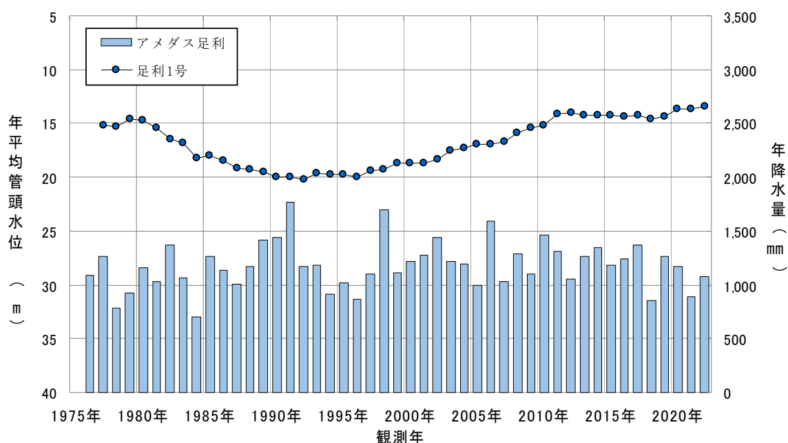
図4.3(25) 年平均地下水位の経年変化（足利1号）
