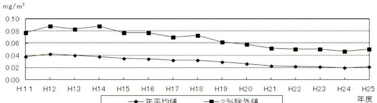
浮遊粒子状物質濃度の推移〔自排局：年平均値・2%除外値〕
