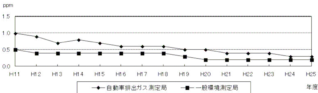
一酸化炭素濃度の推移〔一般局及び自排局：年平均値〕
