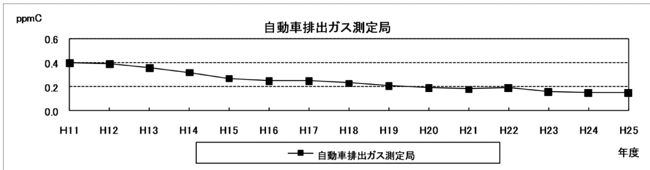
非メタン炭化水素濃度の推移〔自排局：6～9時における年平均値〕
