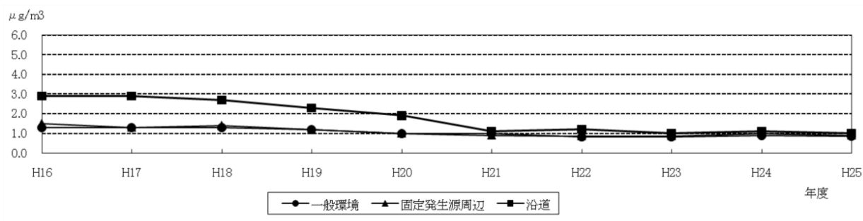
ベンゼン濃度の推移〔年平均値〕
