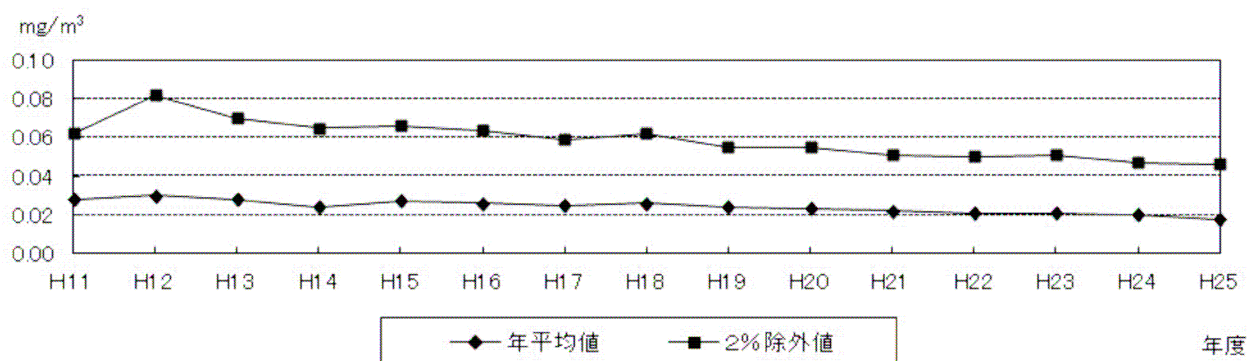
浮遊粒子状物質濃度の推移〔一般局：年平均値・2%除外値〕
