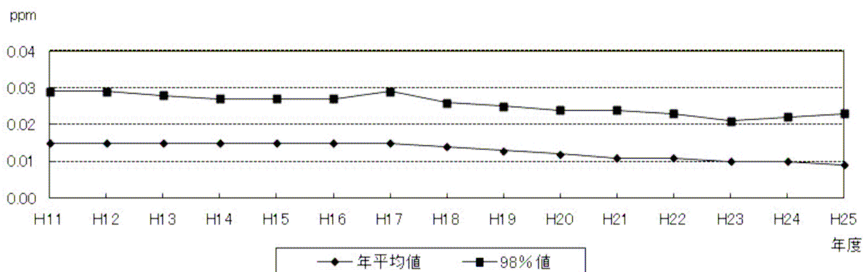
二酸化窒素濃度の推移〔一般局：年平均値・98%値〕
