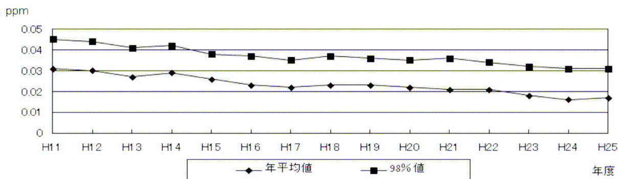
二酸化窒素濃度の推移〔自排局：年平均値・98%値〕
