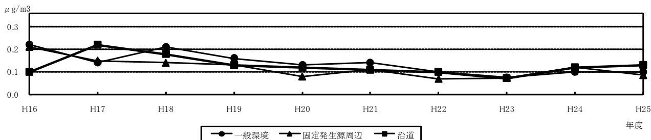
テトラクロロエチレン濃度の推移〔年平均値〕
