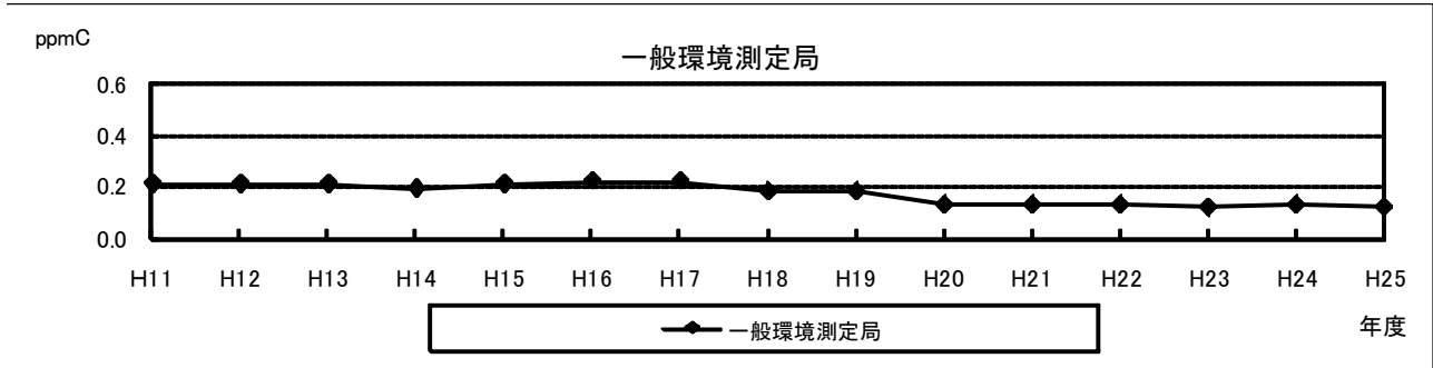
非メタン炭化水素濃度の推移〔一般局：6～9時における年平均値〕
