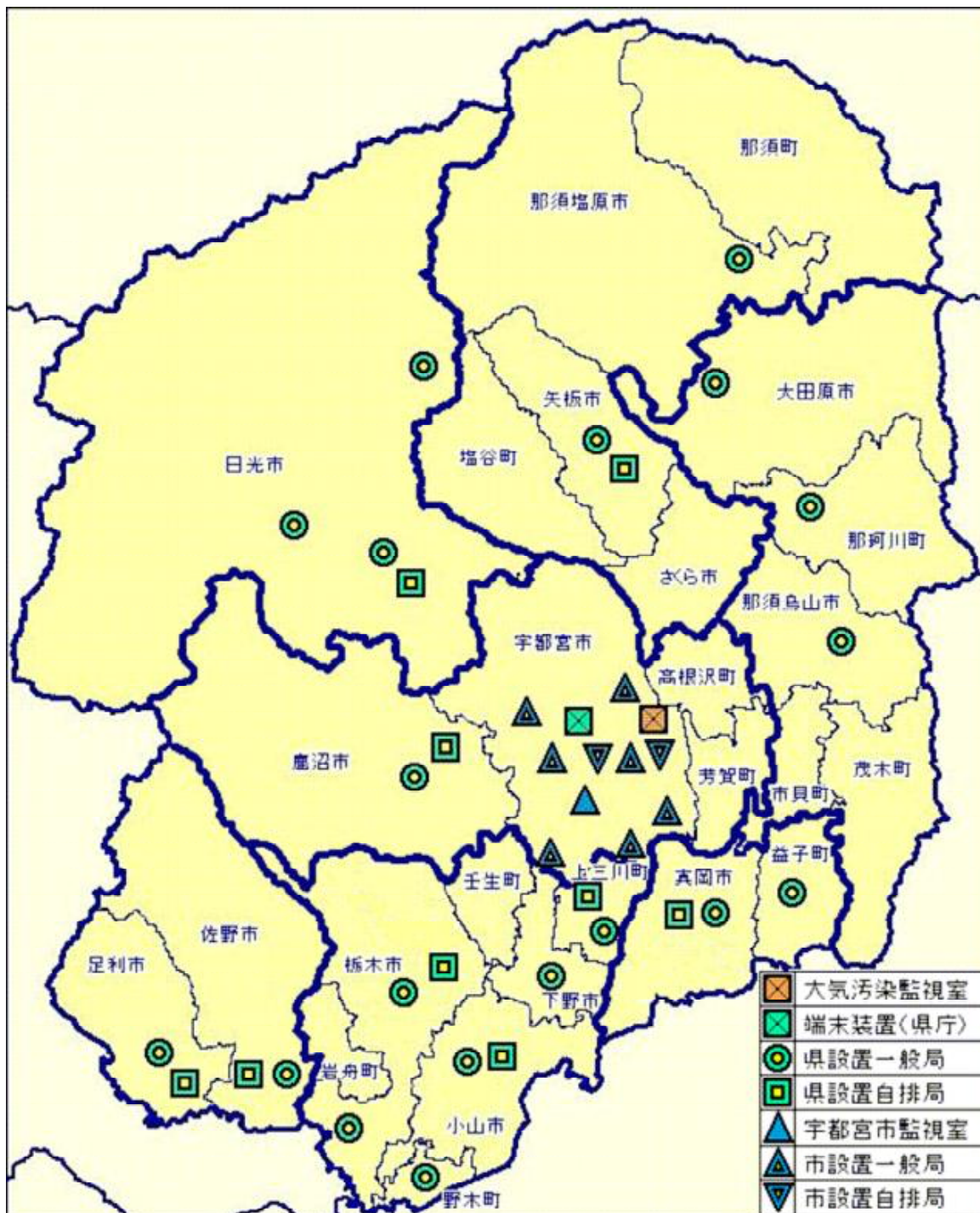
図2-1 大気汚染監視網 (平成26年3月31日現在)
