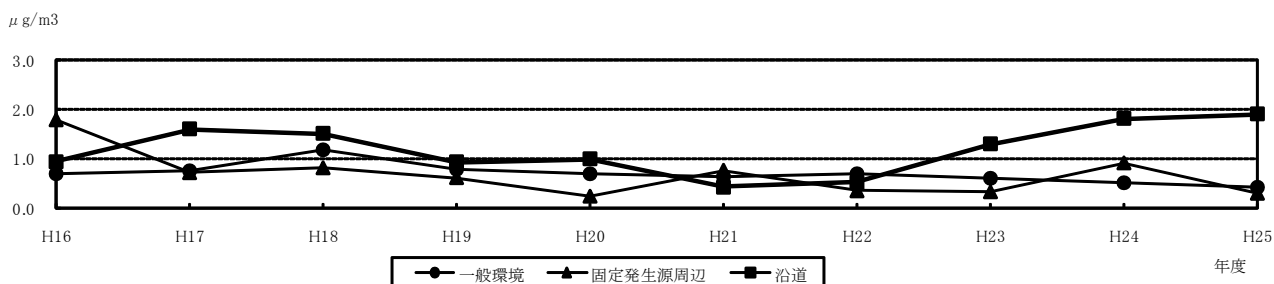
トリクロロエチレン濃度の推移〔年平均値〕
