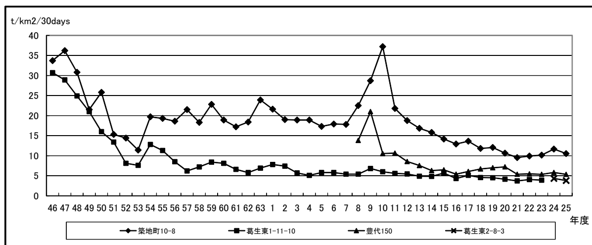
図4-1 佐野市葛生地区における降下ばいじん量の推移〔年平均値〕
