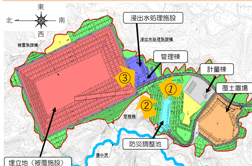
施設配置図
