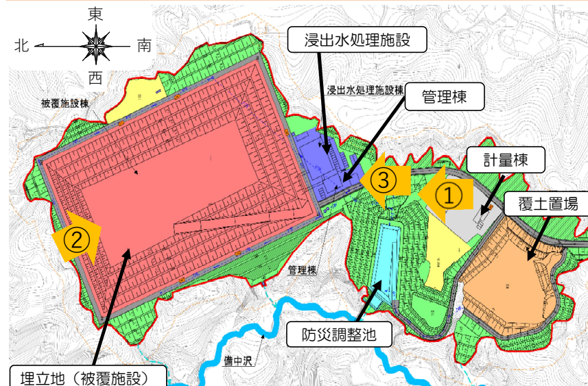
施設配置図
