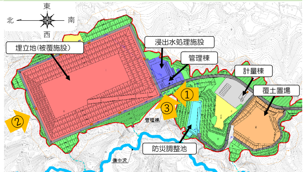
施設配置図
