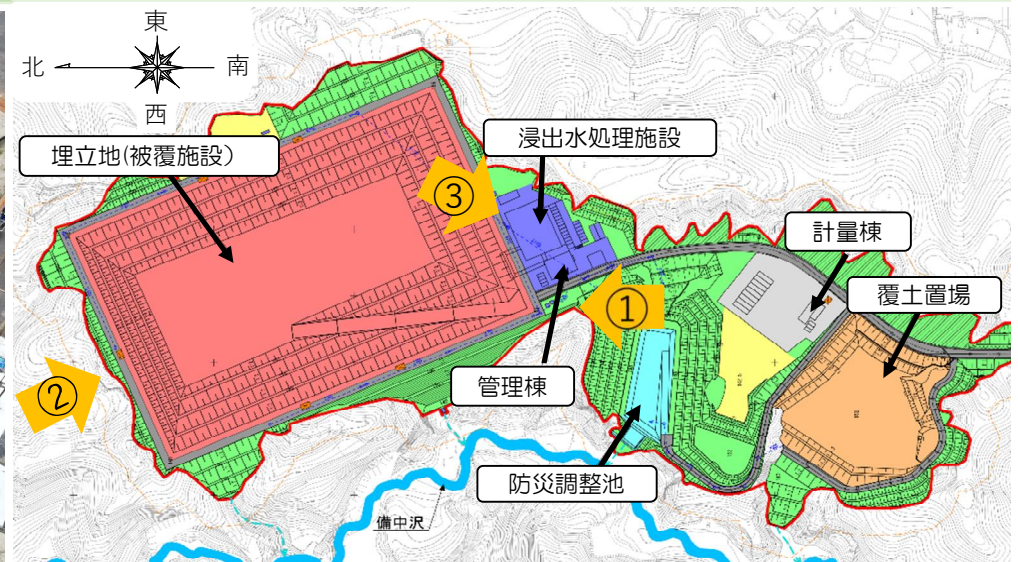
施設配置図
