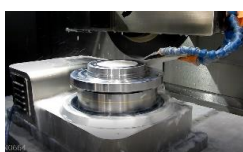
ロータリアタッチメント
