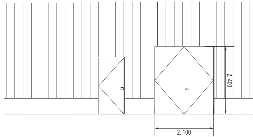
立面図
