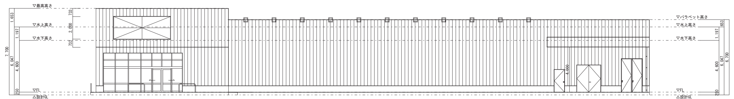
北東側立面図
