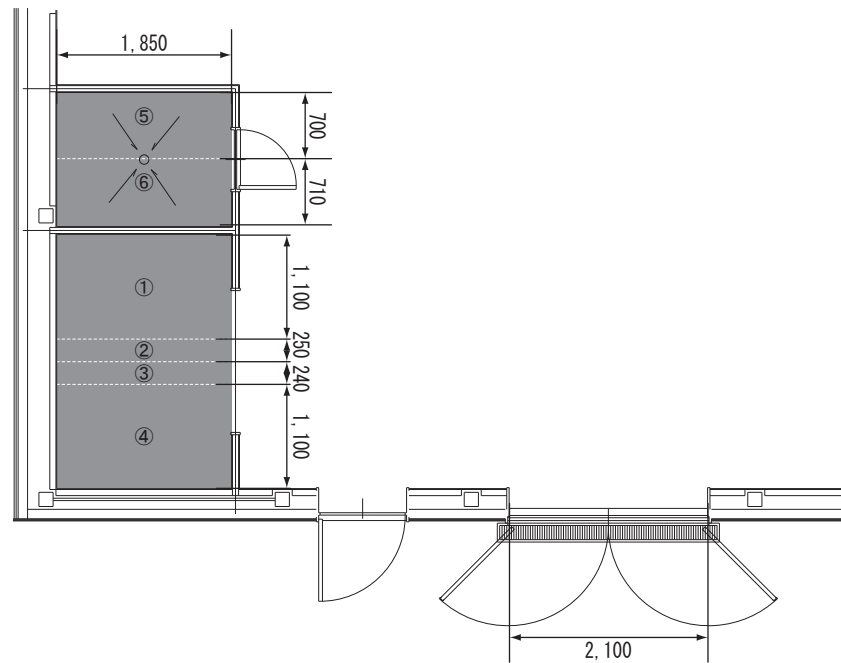
平面図
