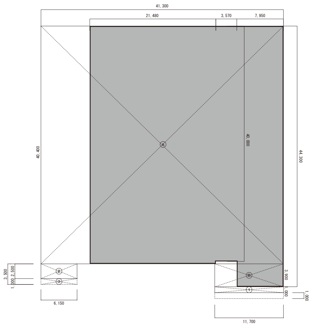
建物求積表
