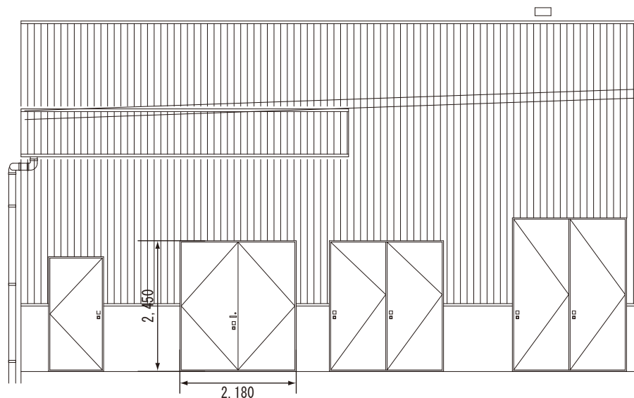
立面図
