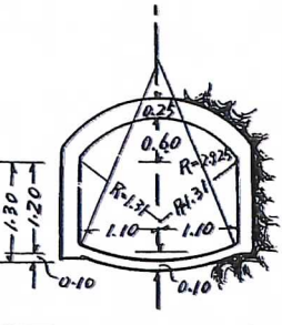
隧道巻立断面 S = \frac{1}{100}
