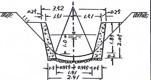
平作堀水路改修標準断面 S = \frac{1}{100}
