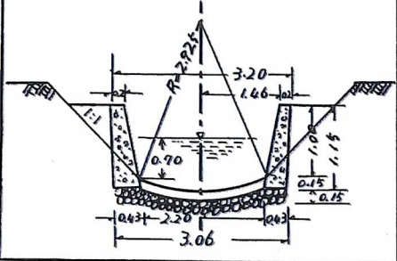
用水幹線ライン標準断面 S = \frac{1}{100}
