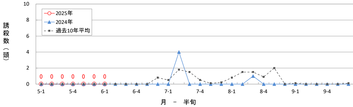
ヒメトビウカの60W予察灯による誘殺数（宇都宮市瓦谷町）
