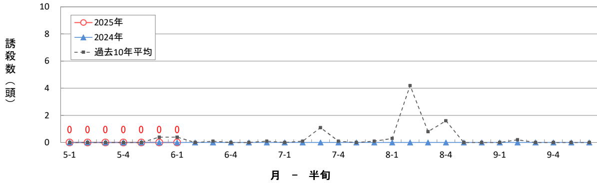
ヒメトビウカの60W予察灯による誘殺数（小山市）
