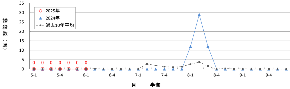
ヒメトビウカの60W予察灯による誘殺数（大田原市）
