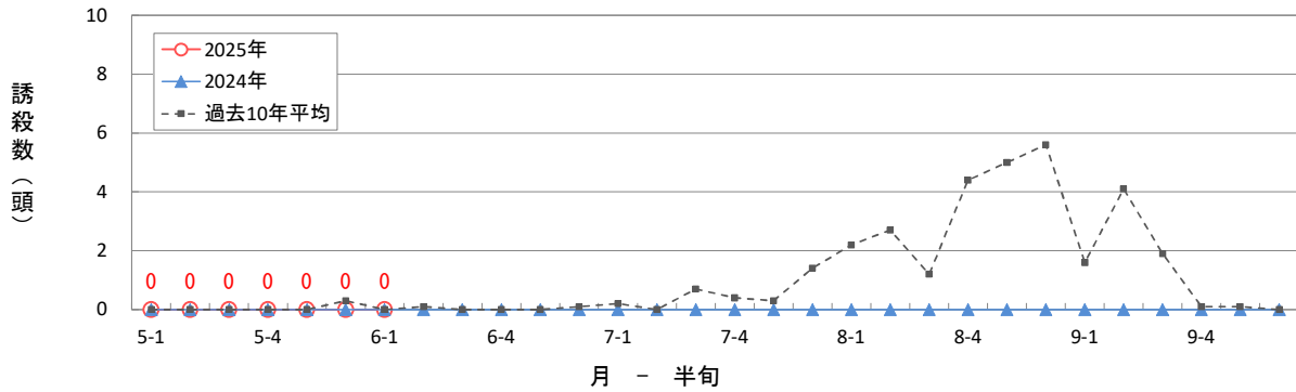
ヒメトビウカの60W予察灯による誘殺数（栃木市大塚町）
