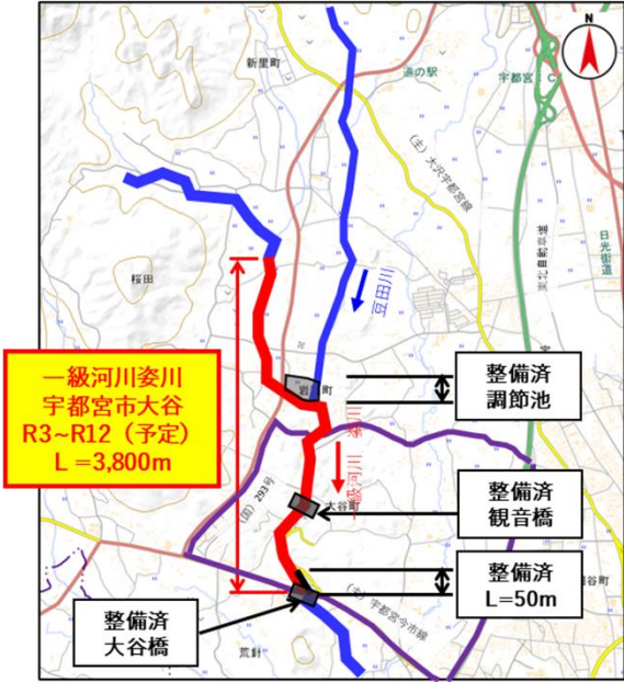
事業平面図
