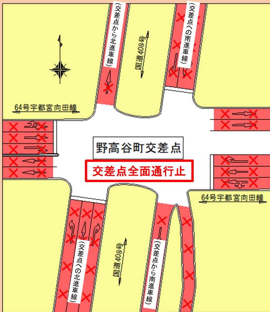
規制図
