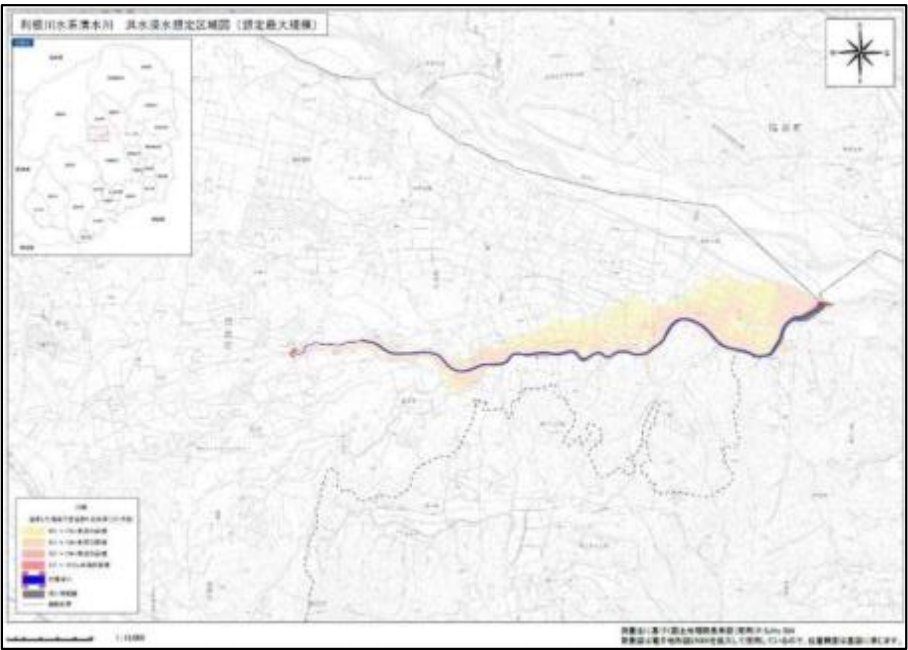
一級河川清水川 洪水浸水想定区域図（日光市）
