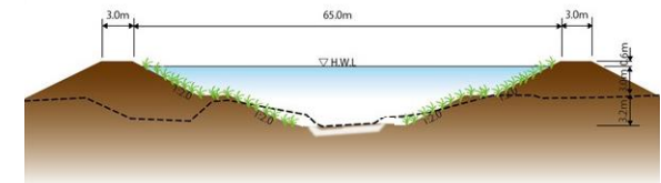
尾名川標準横断面図
