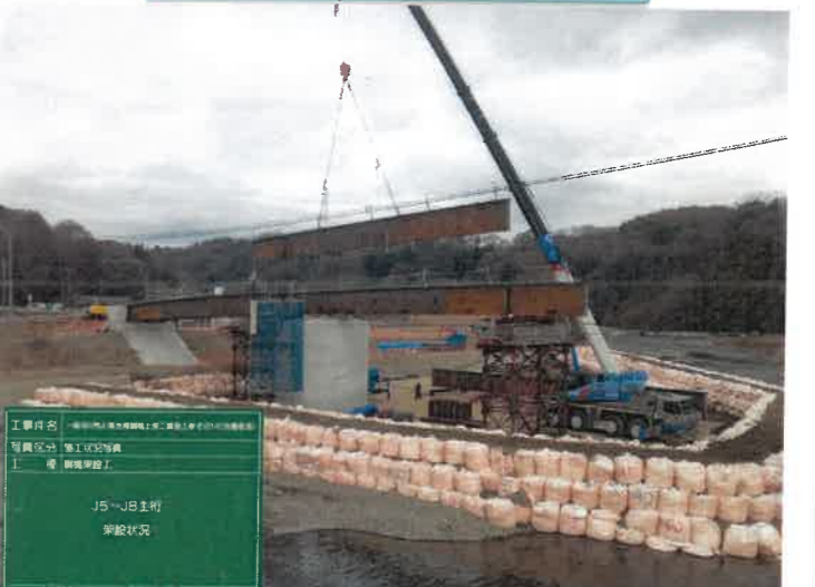
8-1. 桁架設J5~J8
