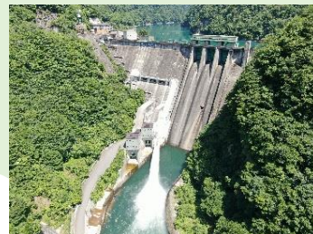
五十里ダム
