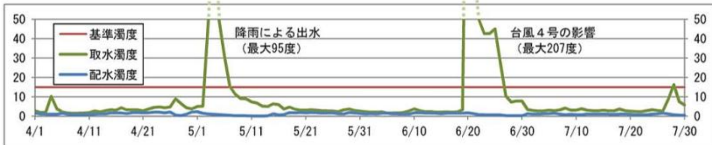
工水配水濁度計
