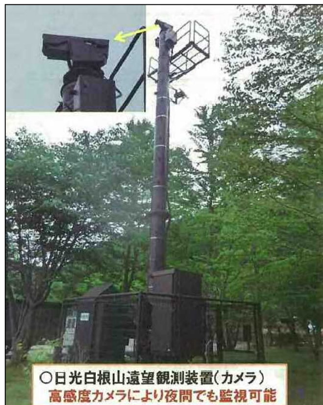
日光白根火山総合観測装置(五色沢設置)
