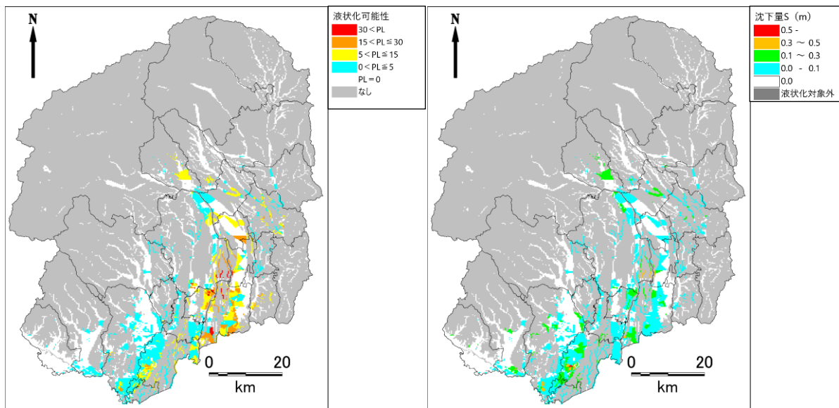
図 2.1-23 液状化危険度（左）・沈下量（右）の予測結果（益子町直下地震）
