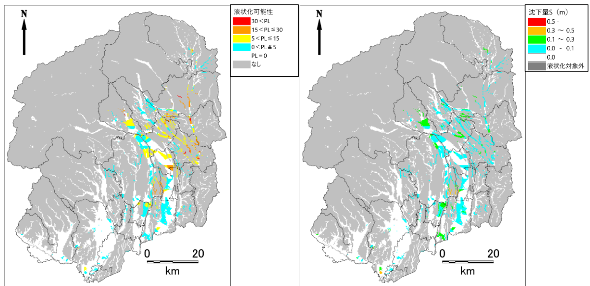
図 2.1-32 液状化危険度（左）・沈下量（右）の予測結果（那珂川町直下地震）
