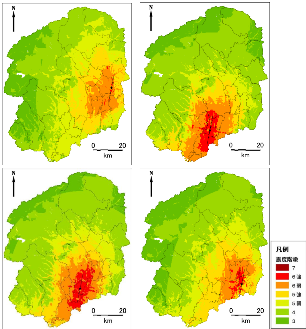
図 2.1-4 各市町直下地震 (M6.9) の地表震度分布図 左上：那須烏山市役所直下地震、右上：下野市役所直下地震 左下：上三川町役場直下地震、右下：益子町役場直下地震 黒星：破壊開始点、線：地表トレース
