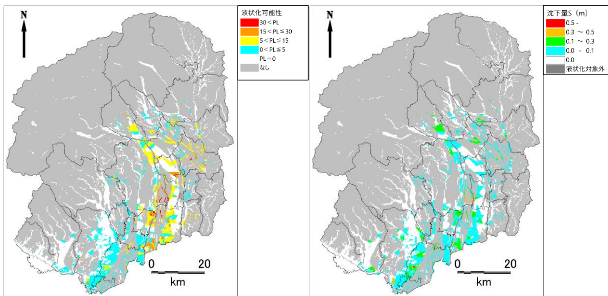
図 2.1-25 液状化危険度（左）・沈下量（右）の予測結果（市貝町直下地震）
