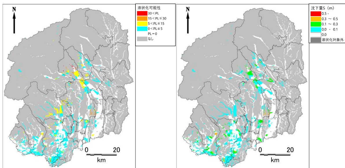
図 2.1-13 液状化危険度（左）・沈下量（右）の予測結果（日光市直下地震）
