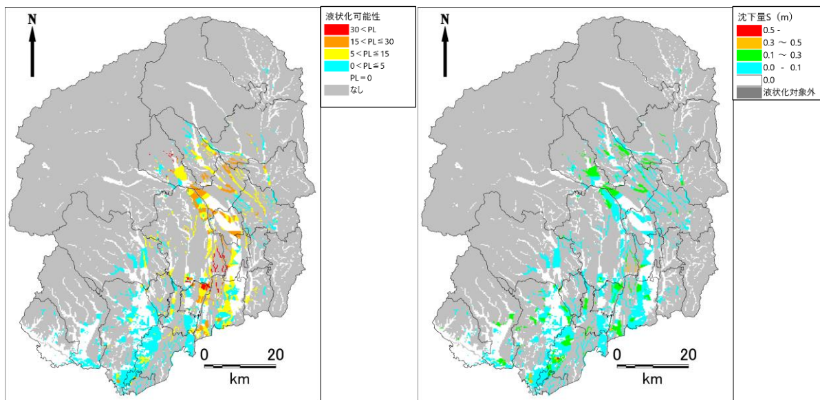
図 2.1-30 液状化危険度（左）・沈下量（右）の予測結果（高根沢町直下地震）
