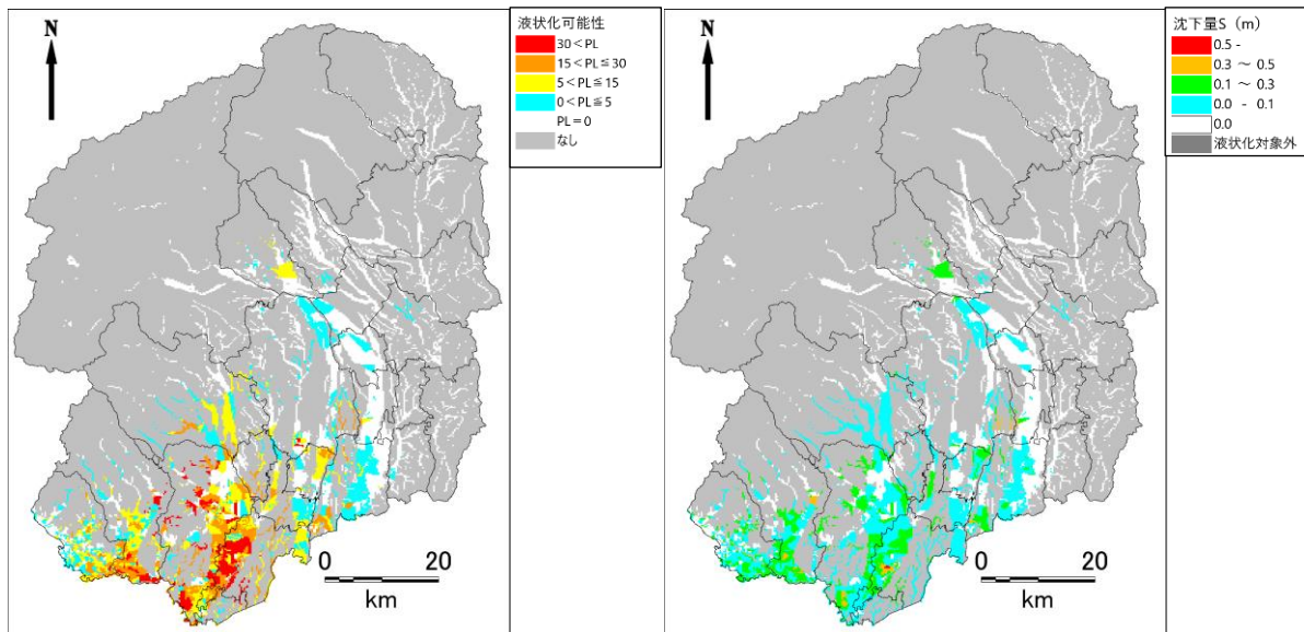
図 2.1-10 液状化危険度（左）・沈下量（右）の予測結果（栃木市直下地震）
