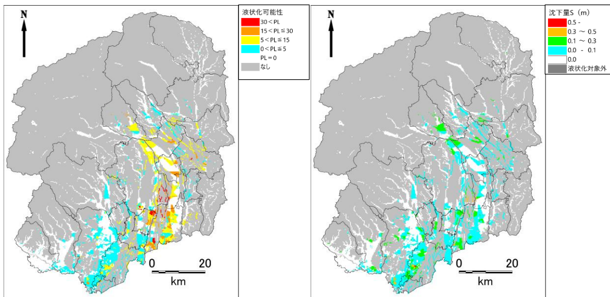
図 2.1-26 液状化危険度（左）・沈下量（右）の予測結果（芳賀町直下地震）
