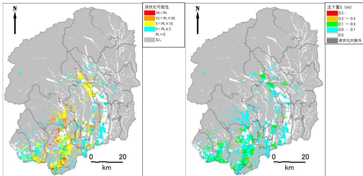
図 2.1-12 液状化危険度（左）・沈下量（右）の予測結果（鹿沼市直下地震）
