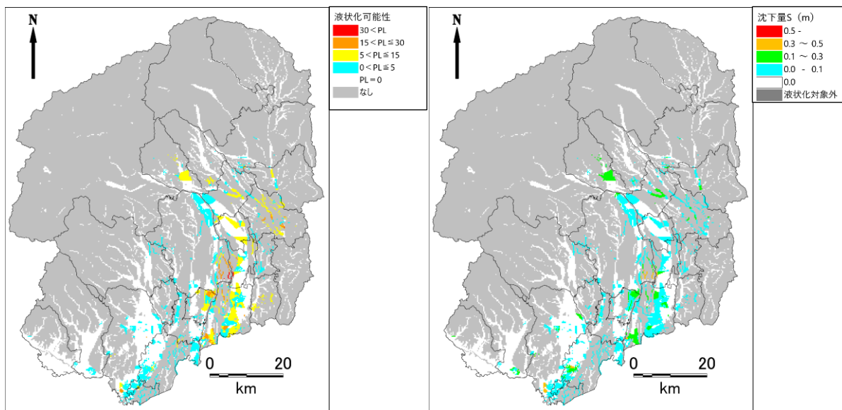
図 2.1-24 液状化危険度（左）・沈下量（右）の予測結果（茂木町直下地震）
