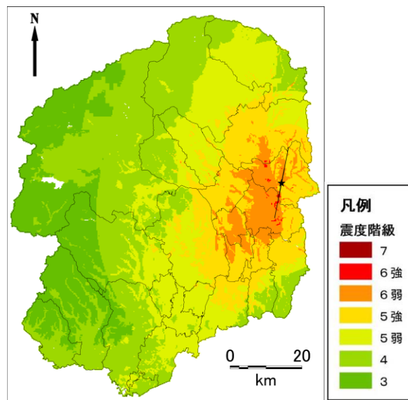
図 2.1-7 各市町直下地震（M6.9）の地表震度分布図 那珂川町役場直下地震 黒星：破壊開始点、線：地表トレース
