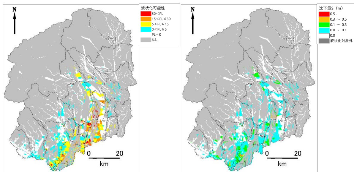
図 2.1-15 液状化危険度（左）・沈下量（右）の予測結果（真岡市直下地震）
