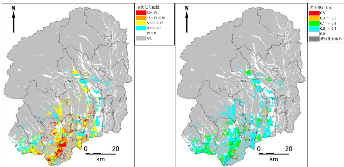
図 2.1-27 液状化危険度（左）・沈下量（右）の予測結果（壬生町直下地震）
