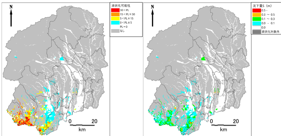
図 2.1-9 液状化危険度（左）・沈下量（右）の予測結果（足利市直下地震）
