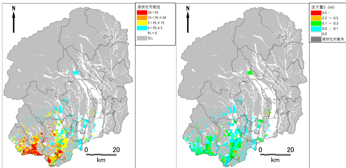
図 2.1-11 液状化危険度（左）・沈下量（右）の予測結果（佐野市直下地震）
