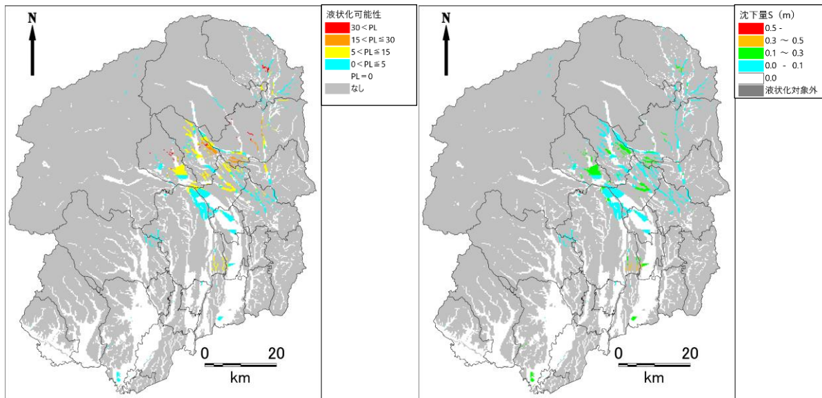
図 2.1-18 液状化危険度（左）・沈下量（右）の予測結果（那須塩原市直下地震）
