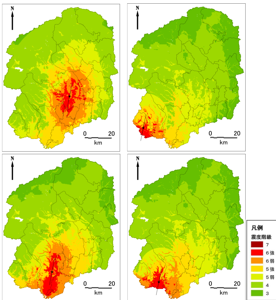
図 2.1-1 各市町直下地震（M6.9）の地表震度分布図 左上：宇都宮市役所直下地震、右上：足利市役所直下地震 左下：栃木市役所直下地震、右下：佐野市役所直下地震 黒星：破壊開始点、線：地表トレース
