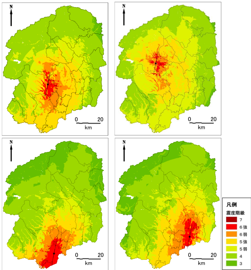
図 2.1-2 各市町直下地震 (M6.9) の地表震度分布図 左上：鹿沼市役所直下地震、右上：日光市役所直下地震 左下：小山市役所直下地震、右下：真岡市役所直下地震 黒星：破壊開始点、線：地表トレース
