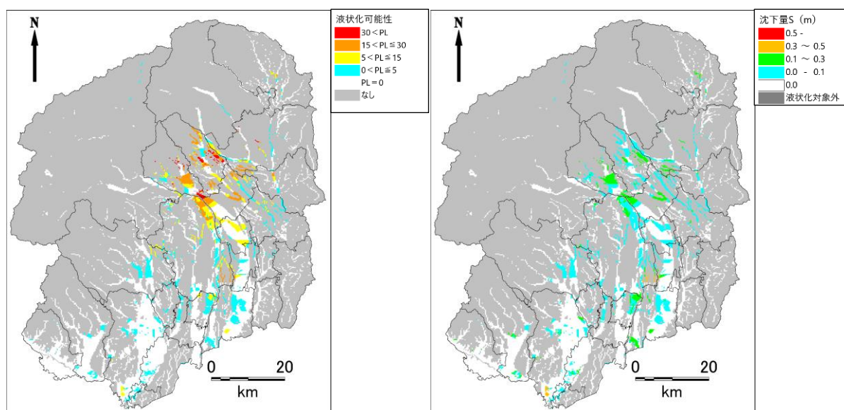
図 2.1-17 液状化危険度（左）・沈下量（右）の予測結果（矢板市直下地震）
