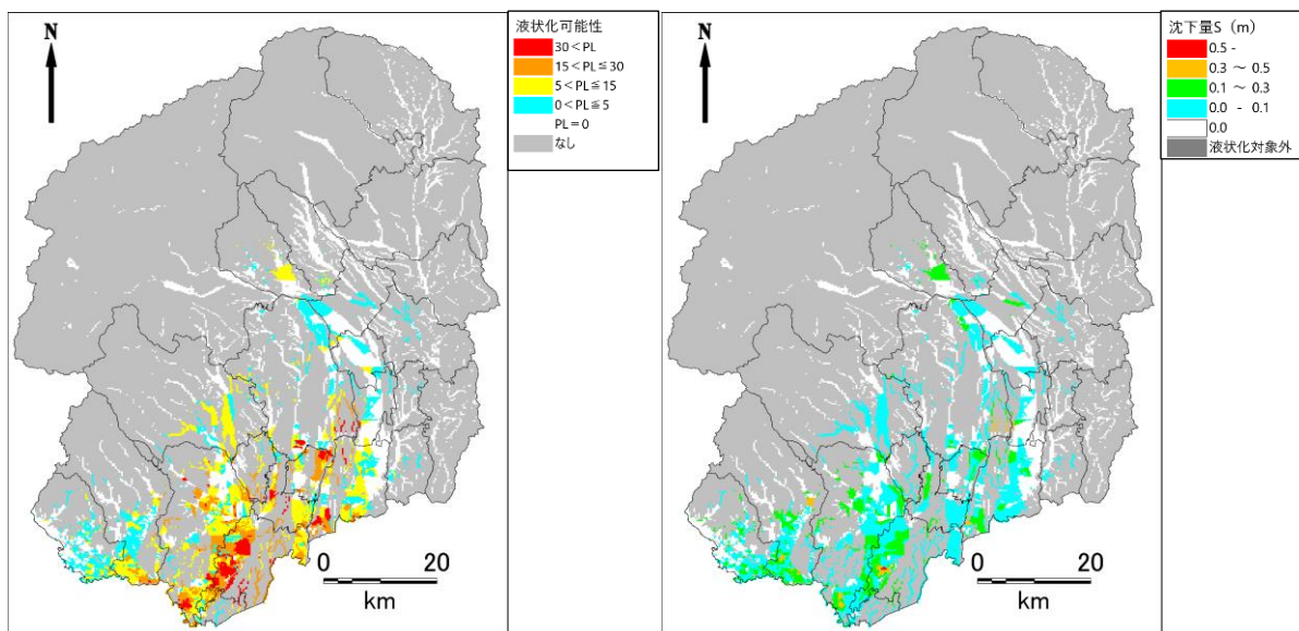
図 2.1-21 液状化危険度（左）・沈下量（右）の予測結果（下野市直下地震）
