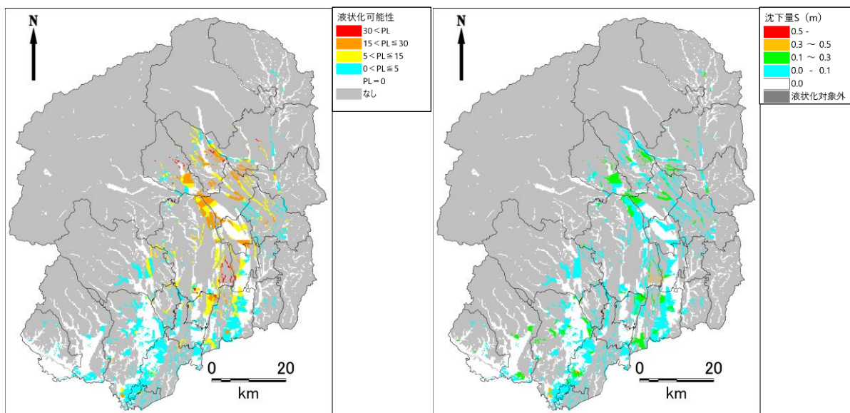
図 2.1-19 液状化危険度（左）・沈下量（右）の予測結果（さくら市直下地震）
