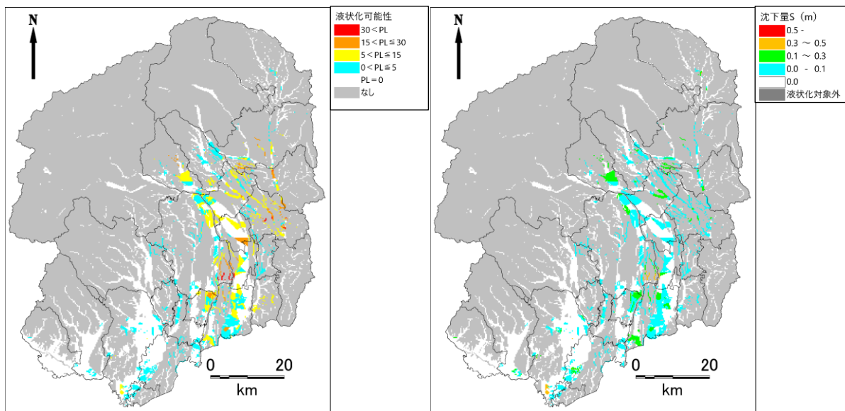
図 2.1-20 液状化危険度（左）・沈下量（右）の予測結果（那須烏山市直下地震）
