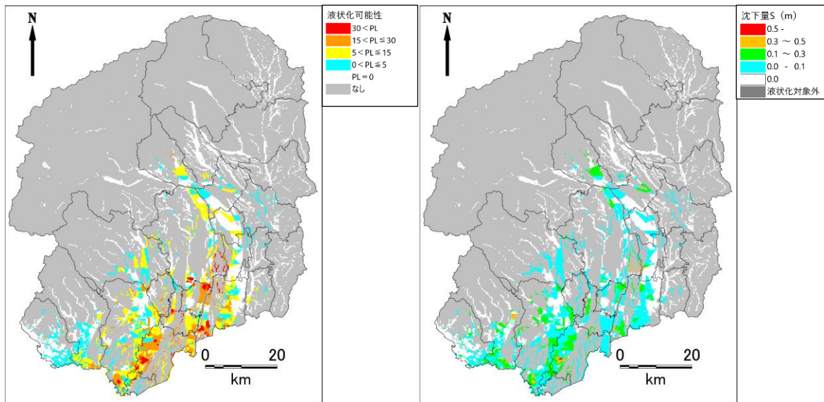
図 2.1-22 液状化危険度（左）・沈下量（右）の予測結果（上三川町直下地震）
