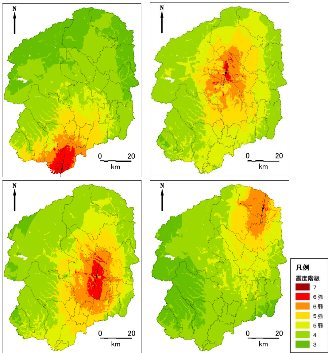
図 2.1-6 各市町直下地震 (M6.9) の地表震度分布図 左上：野木町役場直下地震、右上：塩谷町役場直下地震 左下：高根沢町役場直下地震、右下：那須町役場直下地震 黒星：破壊開始点、線：地表トレース
