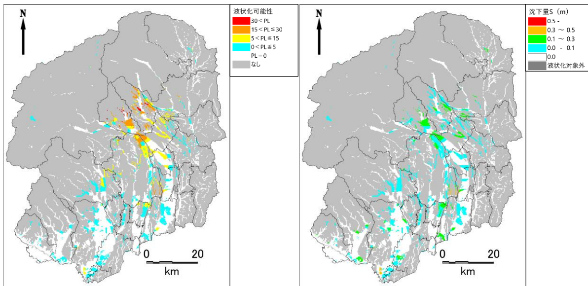
図 2.1-29 液状化危険度（左）・沈下量（右）の予測結果（塩谷町直下地震）
