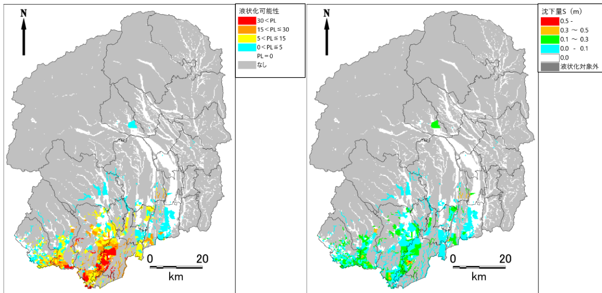
図 2.1-28 液状化危険度（左）・沈下量（右）の予測結果（野木町直下地震）
