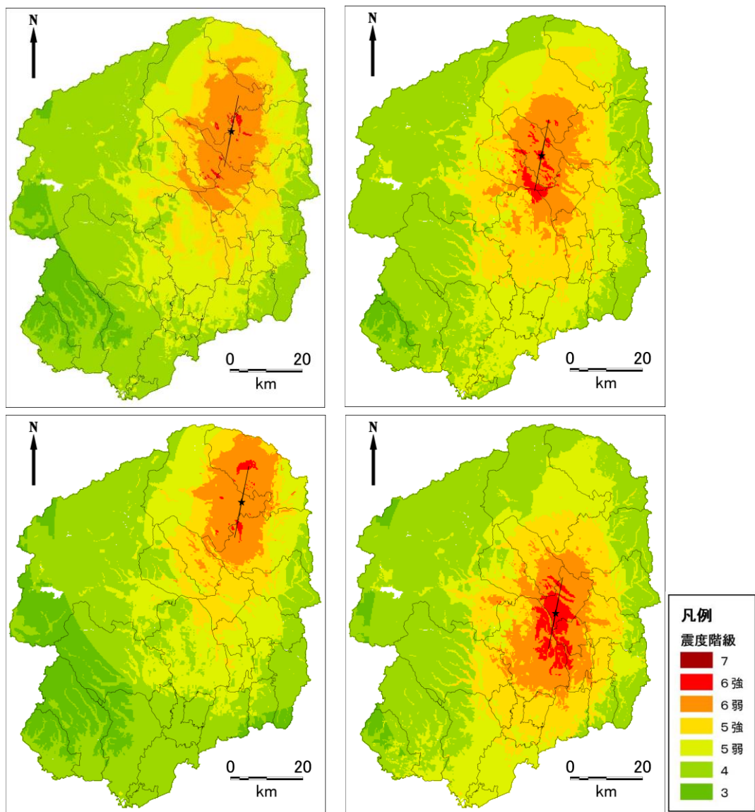
図 2.1-3 各市町直下地震 (M6.9) の地表震度分布図 左上：大田原市役所直下地震、右上：矢坂市役所直下地震 左下：那須塩原市役所直下地震、右下：さくら市役所直下地震 黒星：破壊開始点、線：地表トレース
