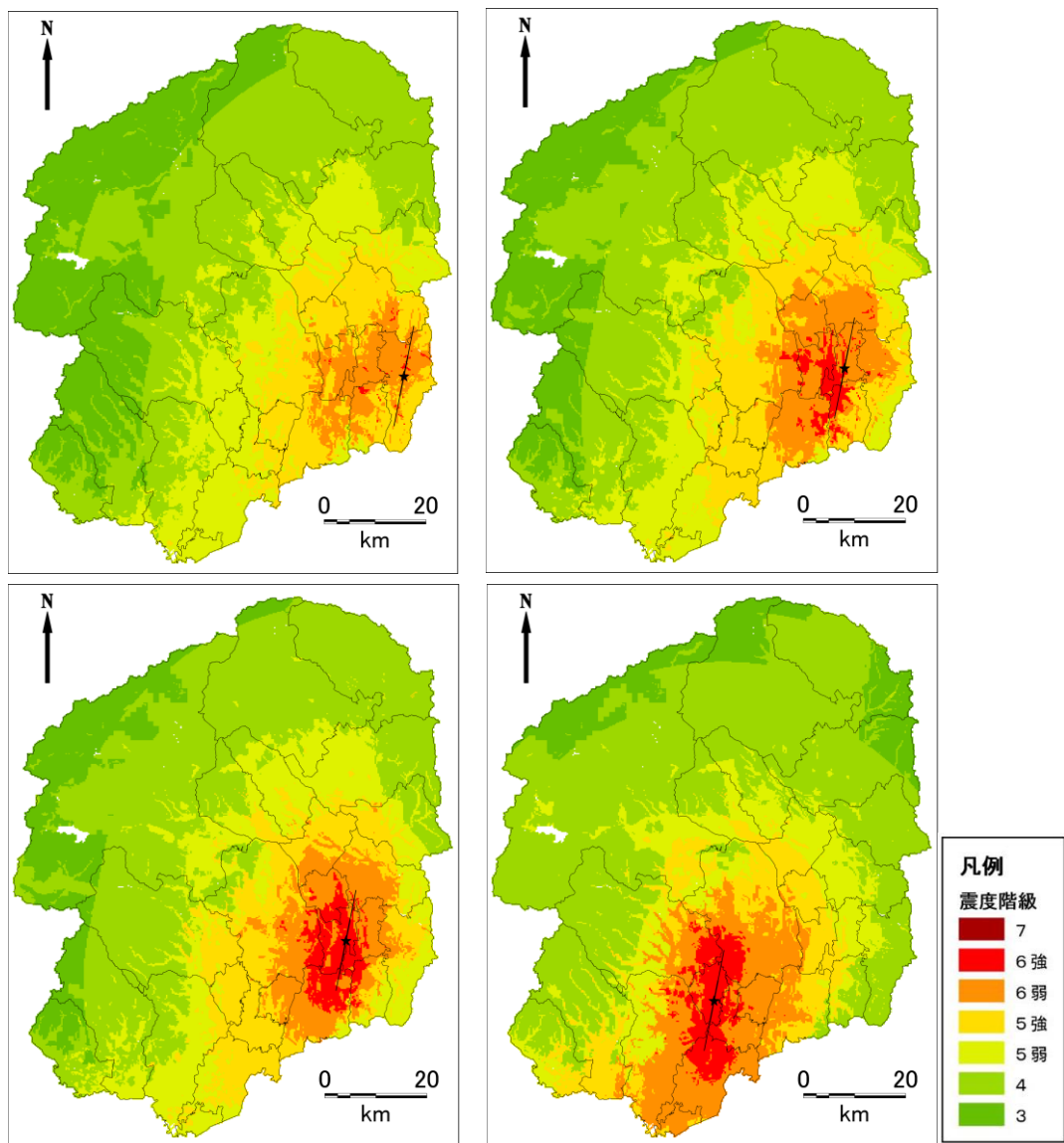
図 2.1-5 各市町直下地震 (M6.9) の地表震度分布図 左上：茂木町役場直下地震、右上：市貝町役場直下地震 左下：芳賀町役場直下地震、右下：壬生町役場直下地震 黒星：破壊開始点、線：地表トレース
