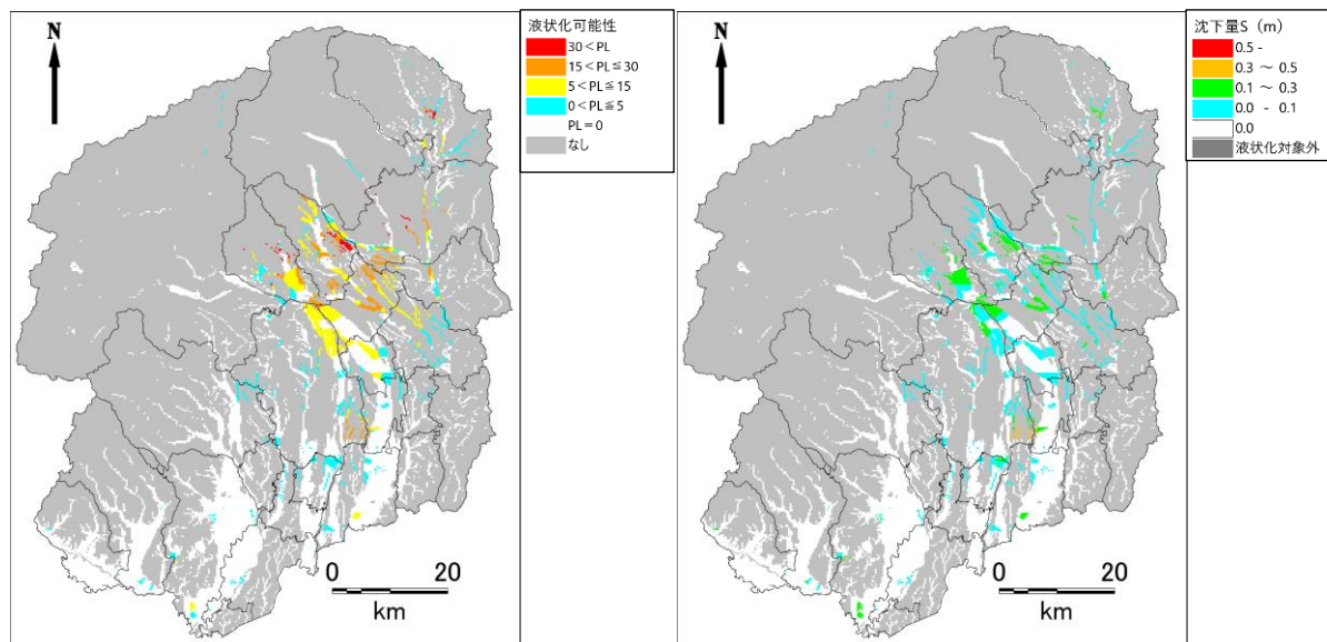
図 2.1-16 液状化危険度（左）・沈下量（右）の予測結果（大田原市直下地震）
