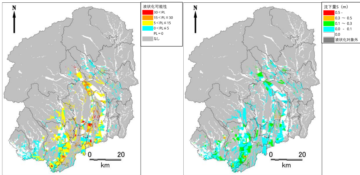
図 2.1-8 液状化危険度（左）・沈下量（右）の予測結果（宇都宮市直下地震）
