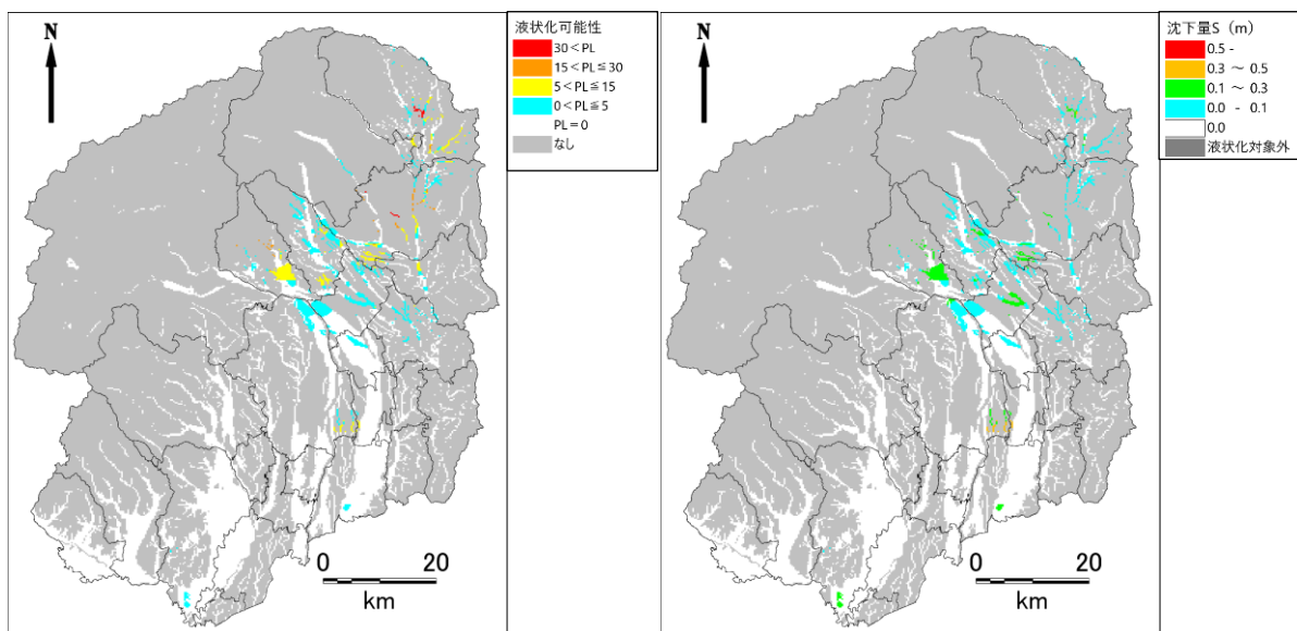
図 2.1-31 液状化危険度（左）・沈下量（右）の予測結果（那須町直下地震）
