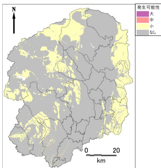
野木町直下地震
