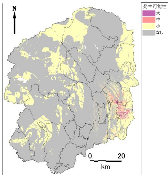
芳賀町直下地震
