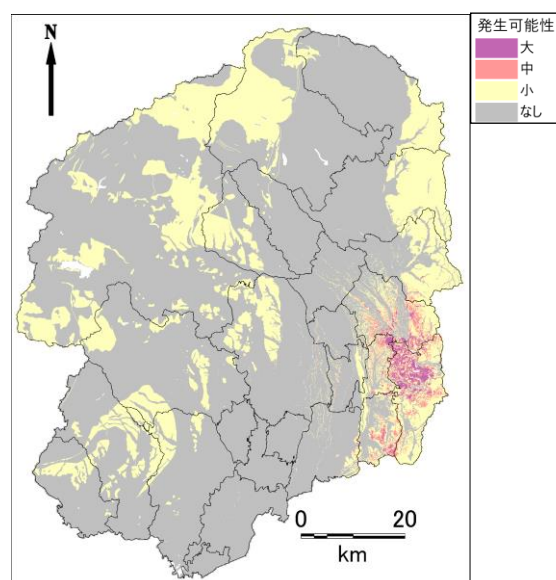
市貝町直下地震
