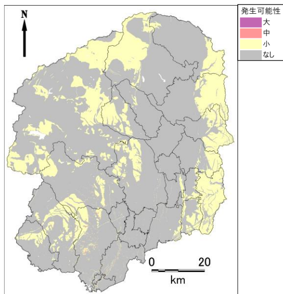
小山市直下地震
