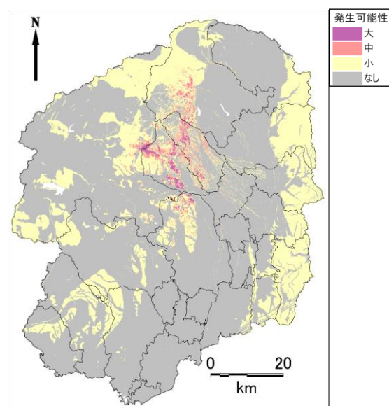
矢板市直下地震
