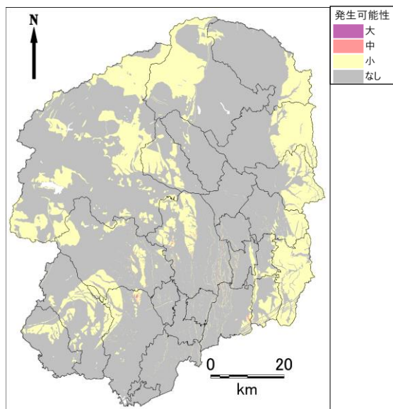
上三川町直下地震
