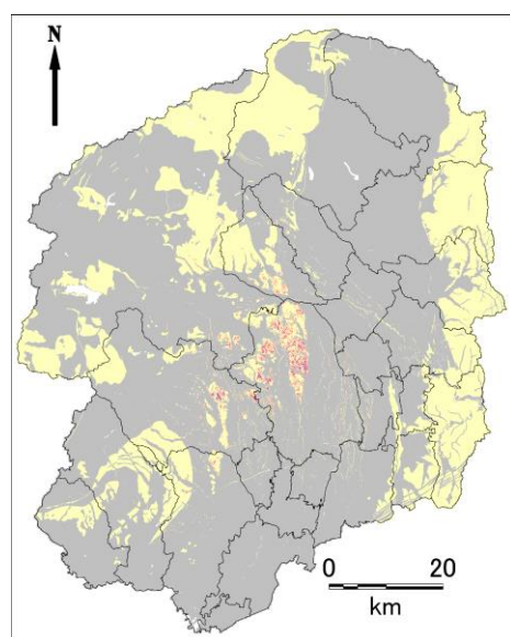
宇都宮市直下地震
