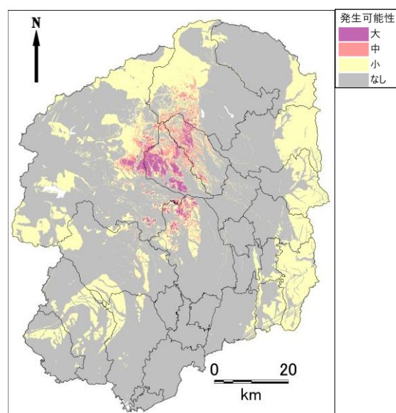
塩谷町直下地震
