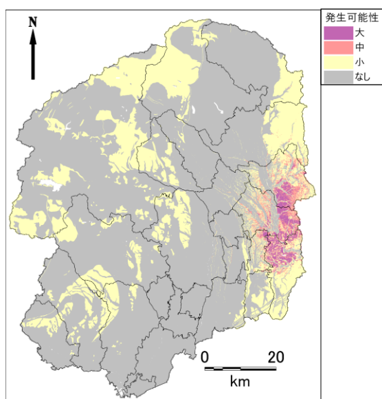
那須烏山市直下地震
