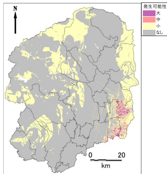
益子町直下地震
