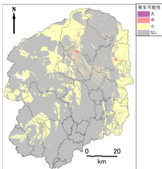
大田原市直下地震
