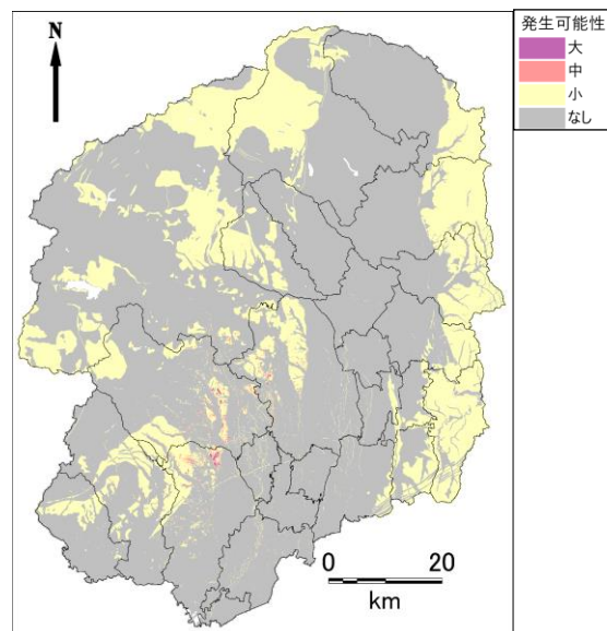
壬生町直下地震
