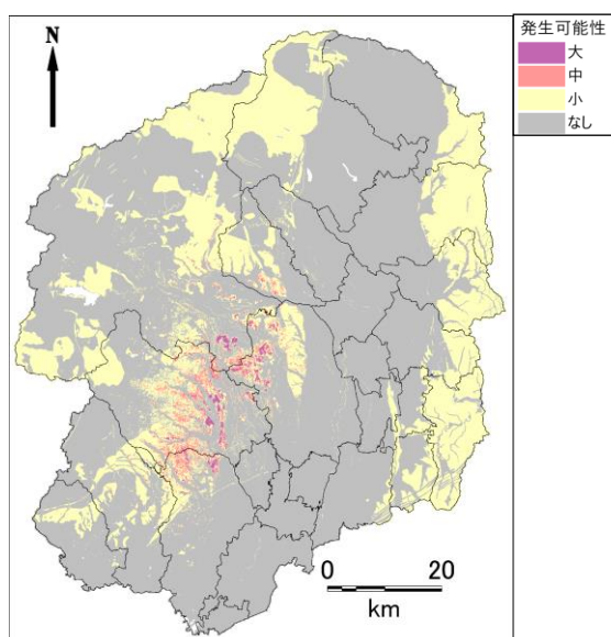
鹿沼市直下地震
