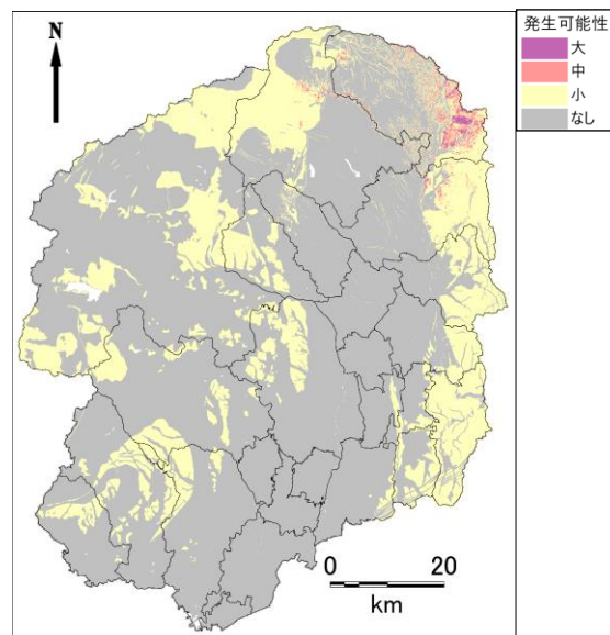
那須町直下地震
