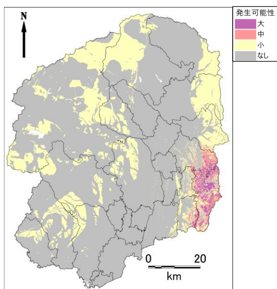
茂木町直下地震
