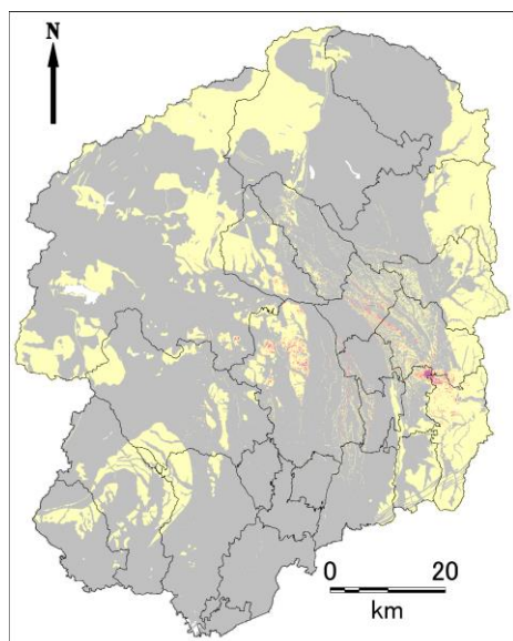
高根沢町直下地震
