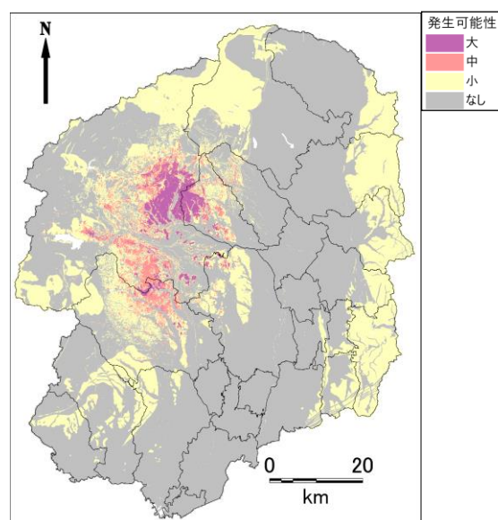
日光市直下地震
