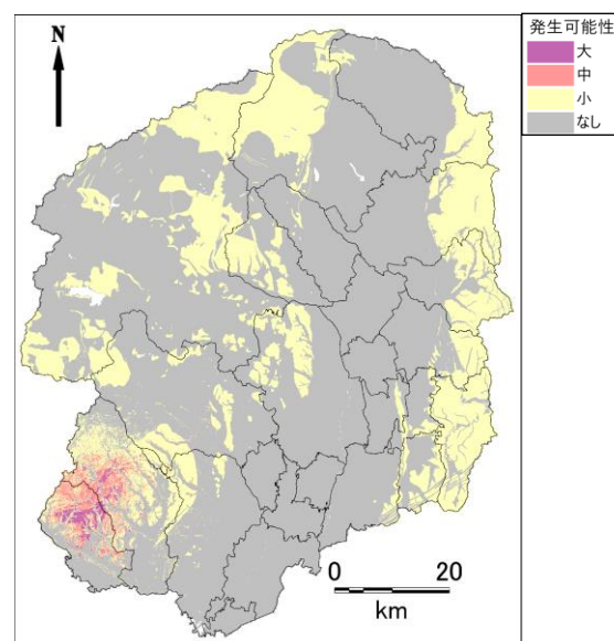
足利市直下地震
