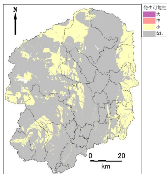
下野市直下地震
