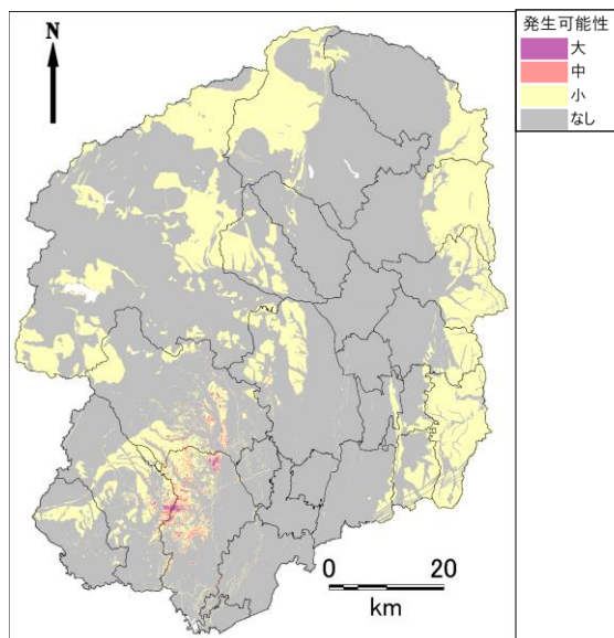
栃木市直下地震
