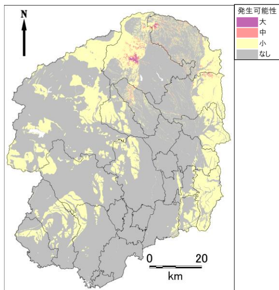
那須塩原市直下地震
