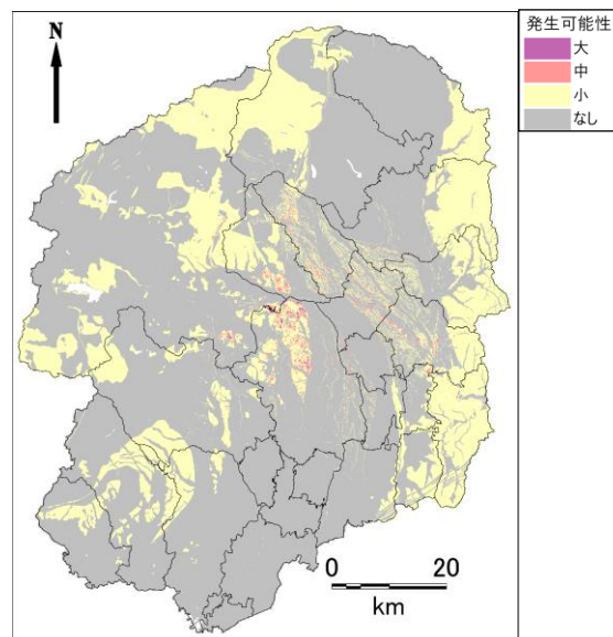
さくら市直下地震
