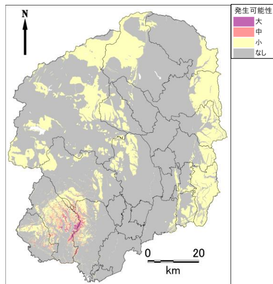
佐野市直下地震
