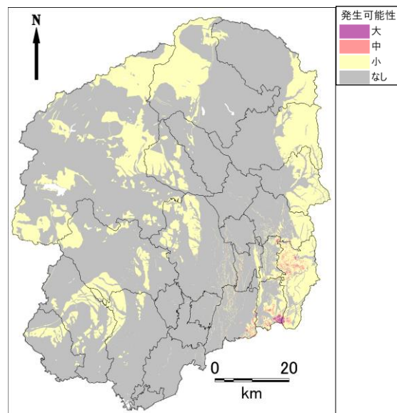
真岡市直下地震
