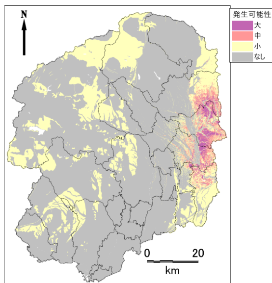
那珂川町直下地震
