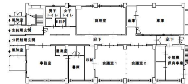
1階平面図
