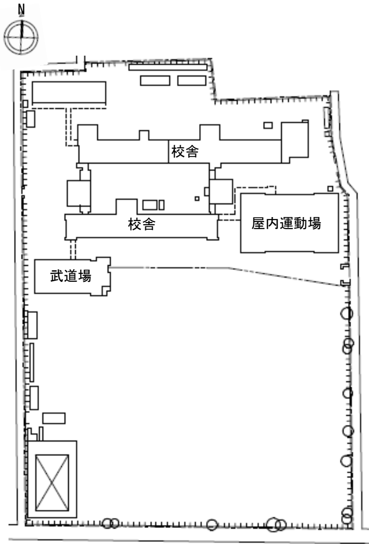
配置図
