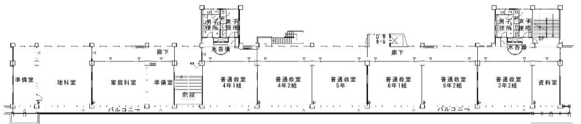
2階平面図
