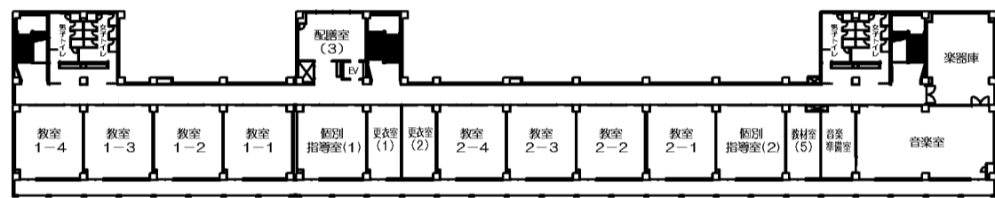
3階平面図
