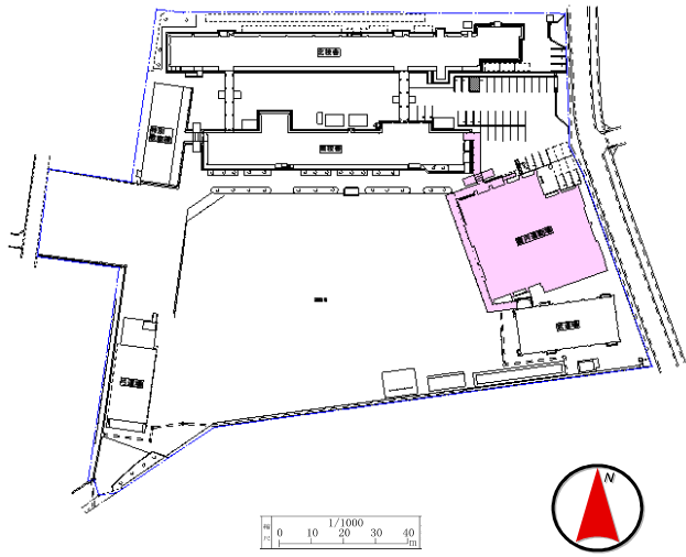
配置図
