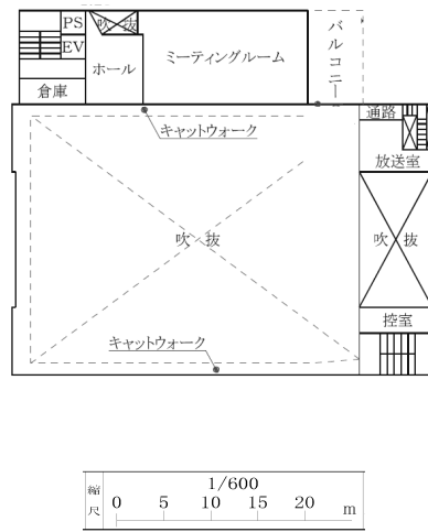
2F 平面図
